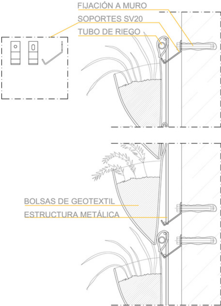
SECCIÓN TIPO
