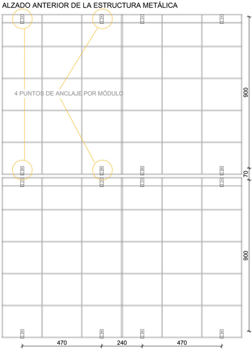
ALZADO DE LA ESTRUCTURA
